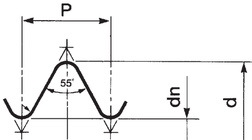
Cilíndrico (ISO 228)
